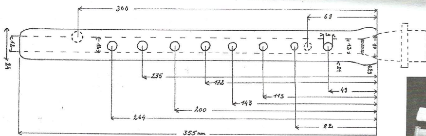
Schéma du duduk B et de son anche
