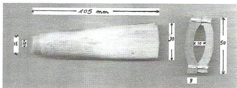
Schéma du duduk B et de son anche
